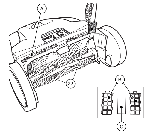
Abb. 8: Staubfilterentnahme
