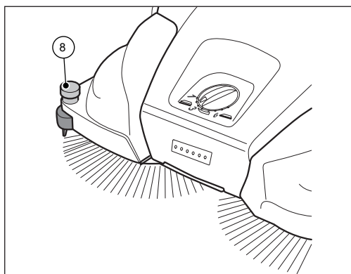
Рис. 6: Установка прижима
