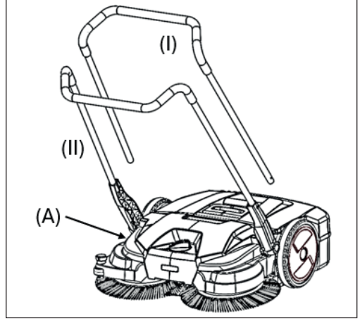
Şek. 3: İtme kolu montajı
