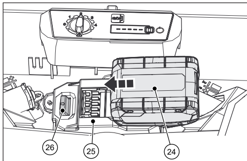
Bild 4: Installera batteri
