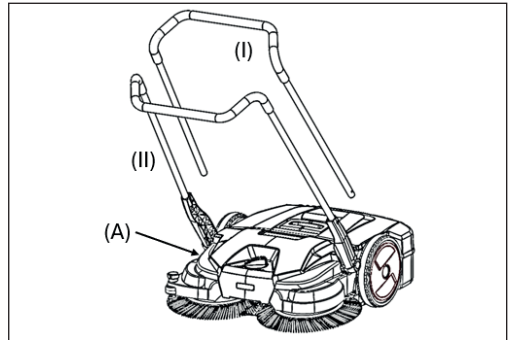
Abb. 3: Schiebebügelmontage
