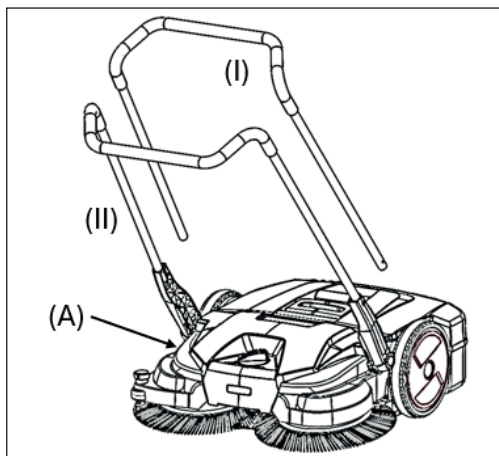
Kuva 3: Työntöaisan kokoaminen
