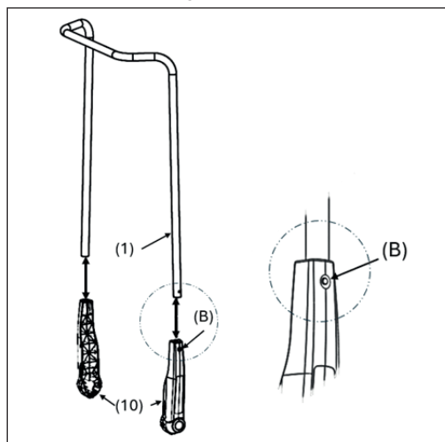
Rys. 2: Montaż uchwytu
