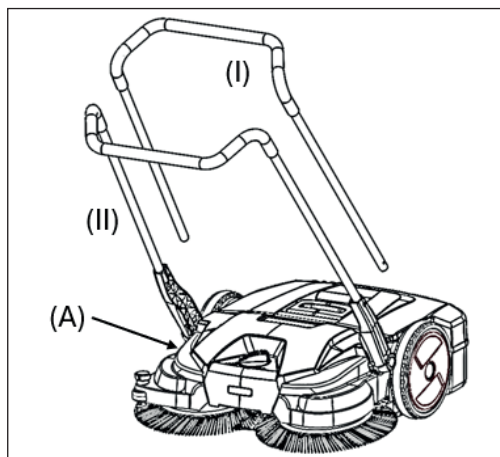
Рис. 3: Монтаж дугообразной ручки
