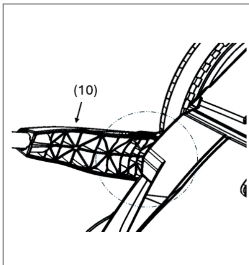
Rys. 9: Demontaż uchwytu do przesuwania
