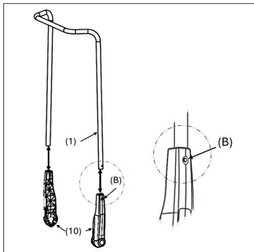
Abb. 2: Monter håndtaksbeslag
