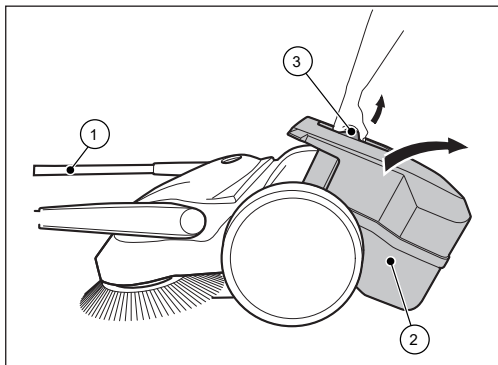
Abb. 7: Tøm oppsamler
