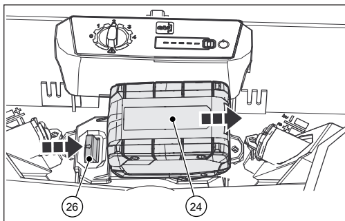
Fig. 10: Retirar la batería
