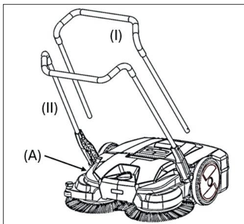
Abb. 3: Montering af skubbebøjlen
