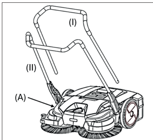
Fig. 3: Montagem do varão de empurrar
