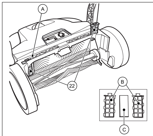
Kuva 8: Pölysuodattimen poistaminen
