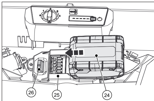
Abb. 4: Akku einbauen
