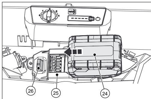
Kuva 4: Akun asennus
