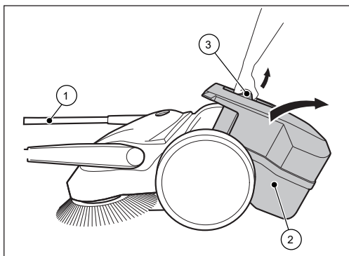
Bild 7: Tömma sopbehållaren
