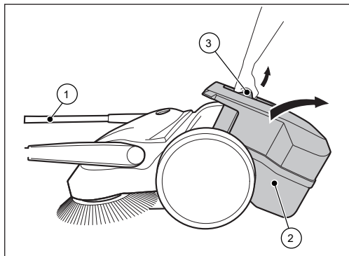
Kuva 7: Säiliön tyhjentäminen
