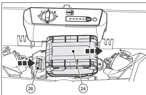
Afb. 10: Accu verwijderen
