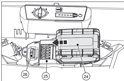
Abb. 4: Sett inn batteri
