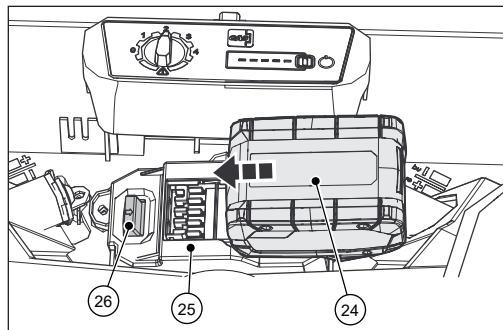
Fig. 4: Montar a bateria
