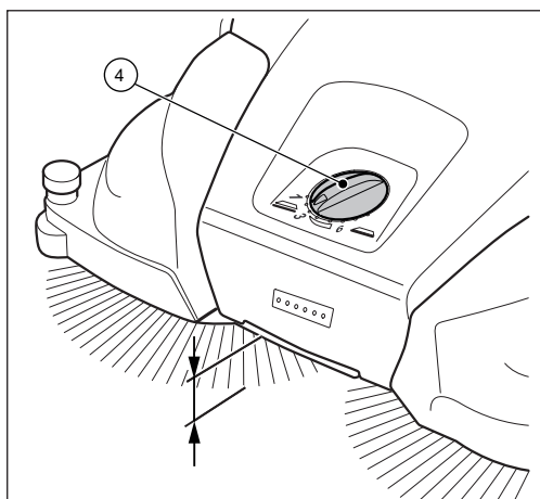
Abb. 5: Höhenverstellung Tellerbesen
