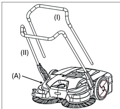
Fig. 3: Montaje del manillar
