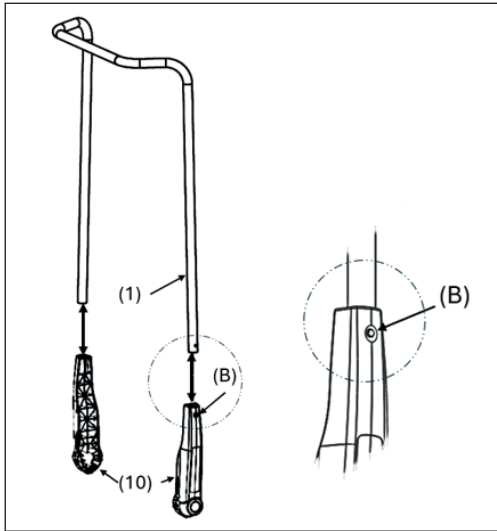
Abb. 2: Griffbeschläge montieren
