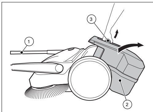
Fig. 7: Vaciado del recipiente recogedor
