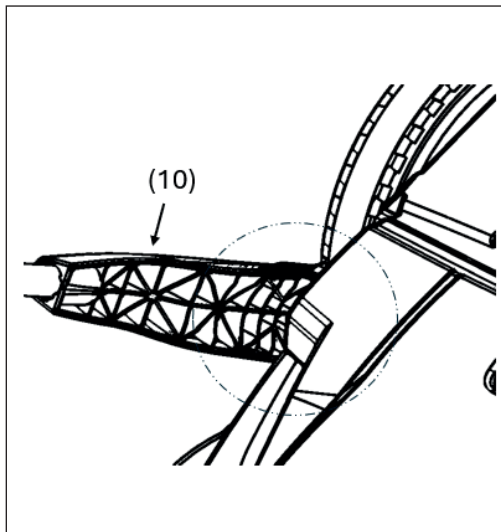
Obr. 9: Demontáž posuvného držadla
