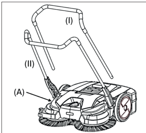
Obr. 3: Montáž posuvného držadla
