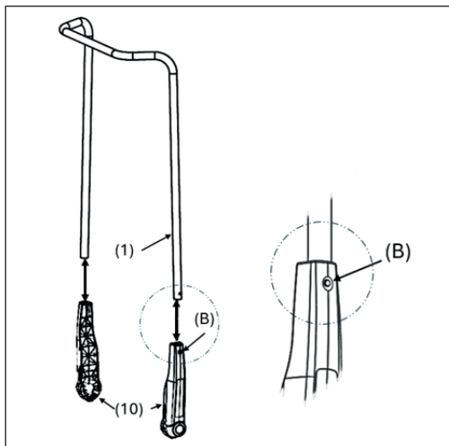
Bild 2: Montera handtagsbeslagen
